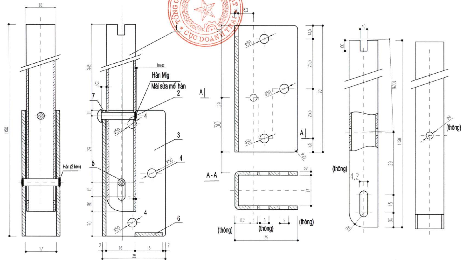
CHI TIẾT CỌC MÀN
