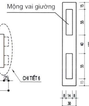
CHI TIẾT 6
