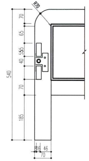
CHI TIẾT 7
