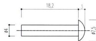
CHI TIẾT CHỐT KHÓA 2
