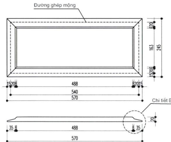
TẤM HUỖNH LỚN
