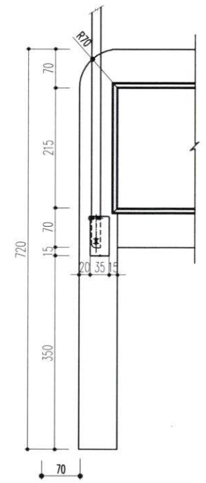
CHI TIẾT 8
