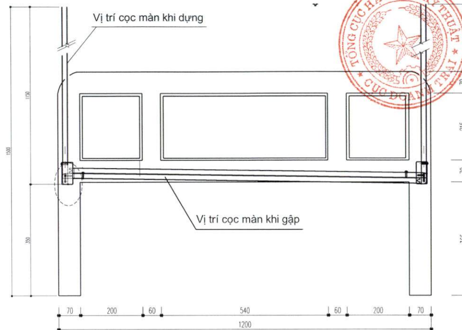
BỐ TRÍ CỌC MÀN ĐẦU CAO
