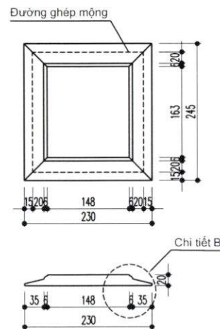
TẤM HUỖNH NHỎ
