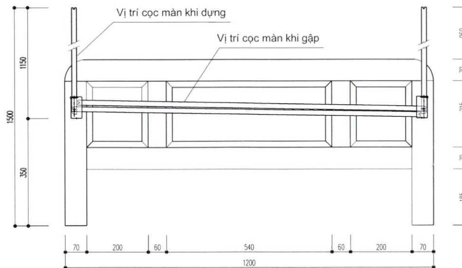
BỐ TRÍ CỌC MÀN ĐẦU THẤP
