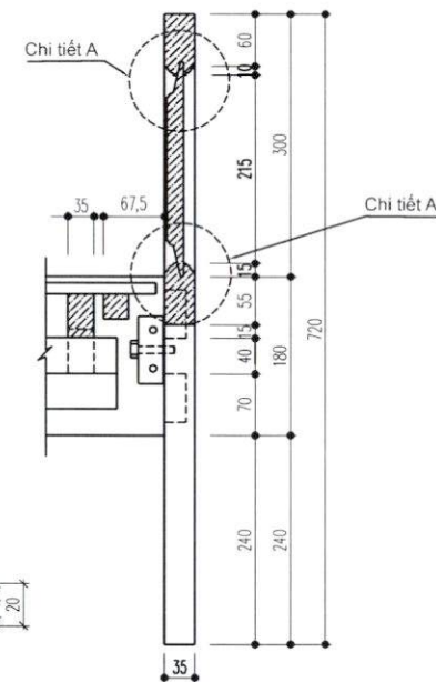
CHI TIẾT 4
