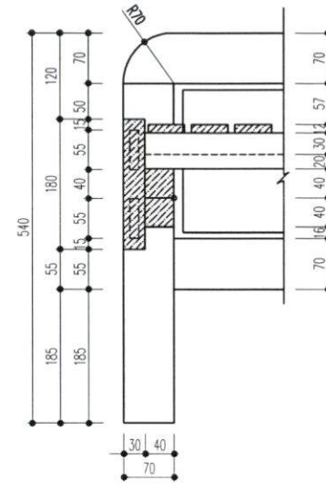
CHI TIẾT 5
